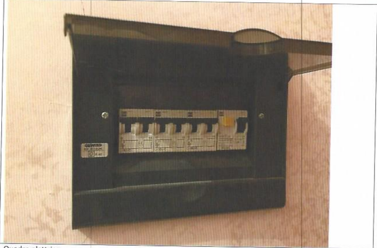
Quadro elettrico
